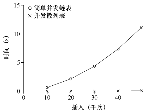
图 29.10 扩展散列表
